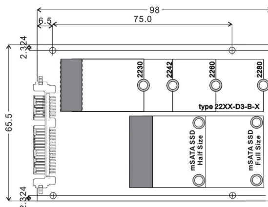
外型尺寸 (单位:mm)
